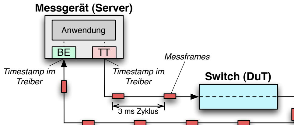
Abbildung 6.5: Hardware-Messung nach Bartols u. a. (2011)
