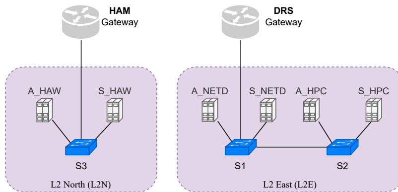
Abbildung 1: Die Layer 2 Netzwerke jeder Gruppe enthalten insgesamt drei Open vSwitches. Jeder Switch spiegelt einen anderen Ort wieder. Die Switches S1 und S3 sind jeweils mit einem Router verbunden (HAM und DRS), welche als Gateways in das größere Netzwerk dienen.
