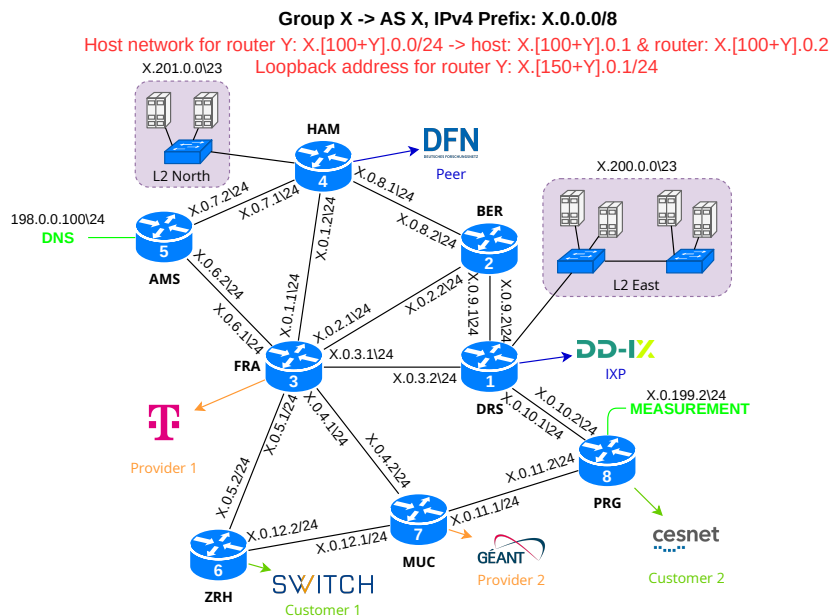
Abbildung 2: Ihr AS besteht aus acht Routern und hat einen /8 IPv4 Präfix, der von ihrer AS Nummer abhängt und für die Konfiguration genutzt wird. Jeder Router ist mit einem Host verbunden. HAM und DRS sind zusätzlich mit den Layer 2 Netzwerken (Abbildung 1) verbunden. Bitte nutzen Sie die hier angegebenen Präfixe für die Konfiguration.
